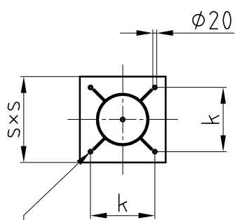
Ankerschraube M16 Qual. St.52 320 mm einbetoniert
