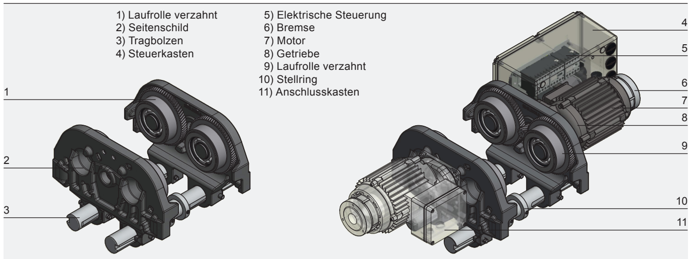
Abbildung 1-2 GHF 5000/6300 und GMF 4000/5000/6300
